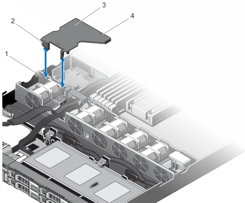
Abbildung 58. Abdeckung für die Stromverteilungsplatine entfernen und installieren
