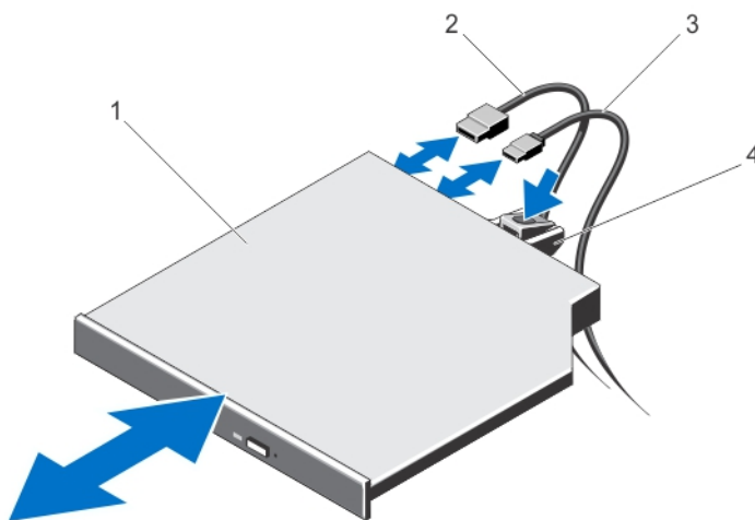
Abbildung 26. Optisches Laufwerk entfernen und installieren (Systeme mit hot-swap-fähigen Festplatten)
