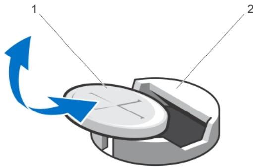
Abbildung 43. Systembatterie austauschen
