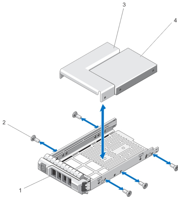
Abbildung 24. Festplattenadapter mit hot-swap-fähiger 2,5-Zoll-Festplatte aus einem 3,5-Zoll-Laufwerkträger entfernen und in einem 3,5-Zoll-Laufwerkträger installieren
