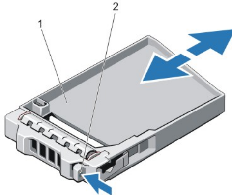
Abbildung 18. 2,5-Zoll-Laufwerkplatzhalter entfernen und installieren
