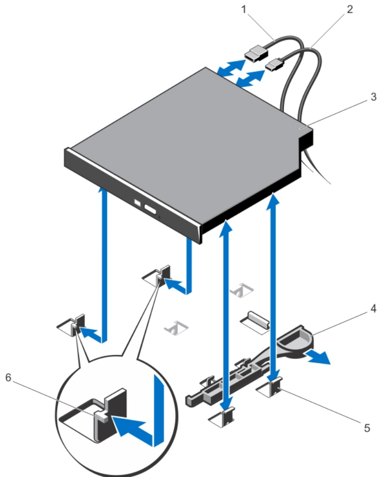
Abbildung 27. Optisches Laufwerk entfernen und installieren (Systeme mit verkabelten Festplatten)
