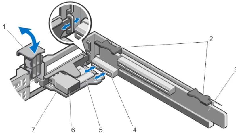
Abbildung 34. iDRAC-Port-Karte entfernen und installieren
