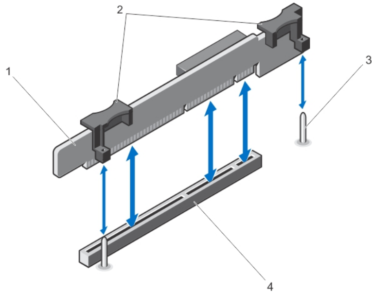
Abbildung 32. Erweiterungskarten-Riser 1 entfernen und installieren
