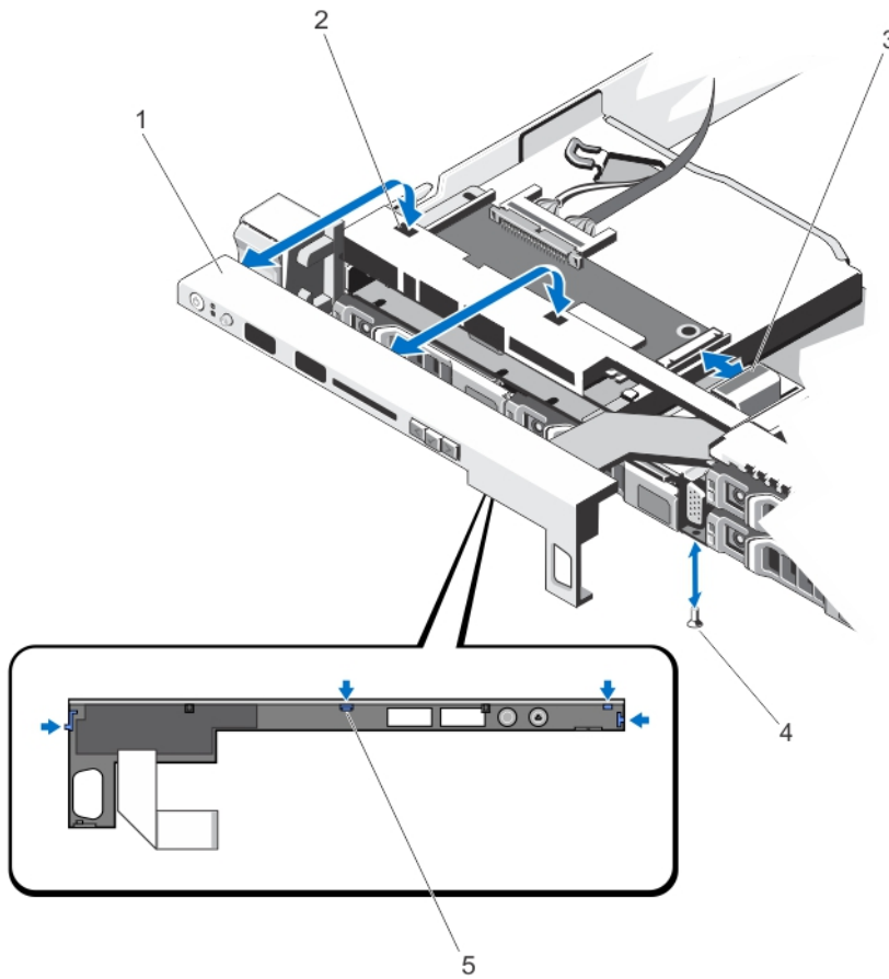
Abbildung 53. Bedienfeld entfernen und installieren – System mit acht Festplatten
