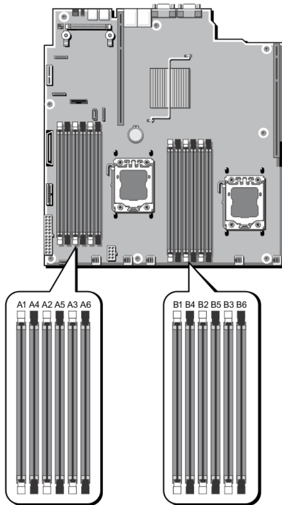
Abbildung 14. Positionen der Speichersockel
