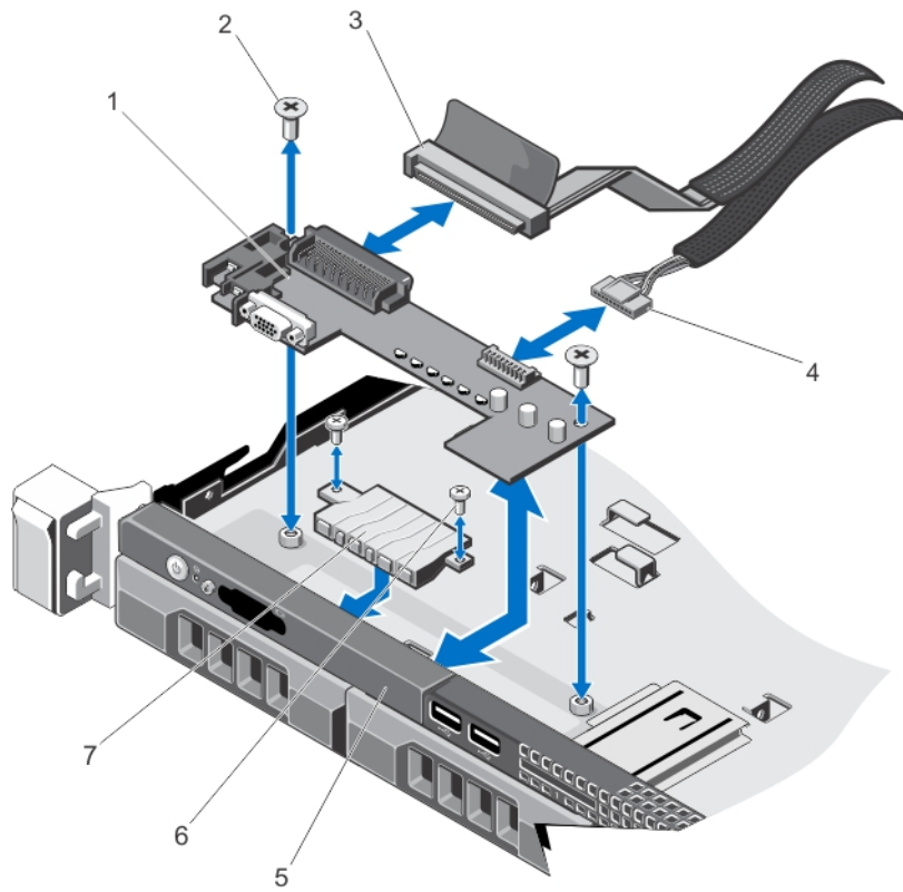
Abbildung 54. Bedienfeldmodul entfernen und installieren – System mit verkabelten 3,5-Zoll-Festplatten
