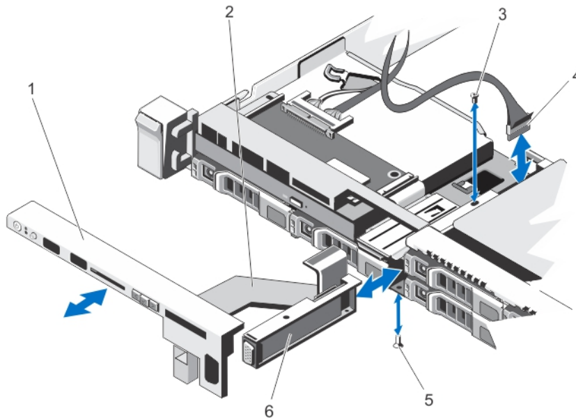
Abbildung 57. VGA-Modul entfernen und installieren
