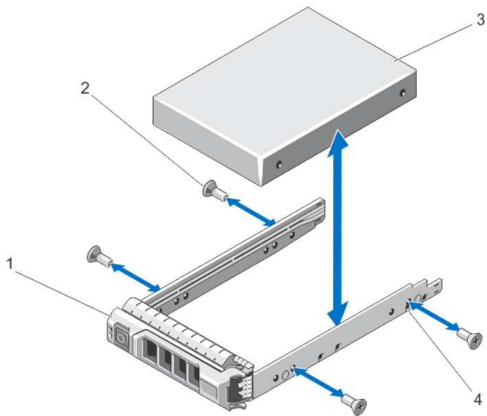
Abbildung 23. Hot-swap-fähige Festplatte aus einem Laufwerkträger entfernen und in einem Laufwerkträger installieren
