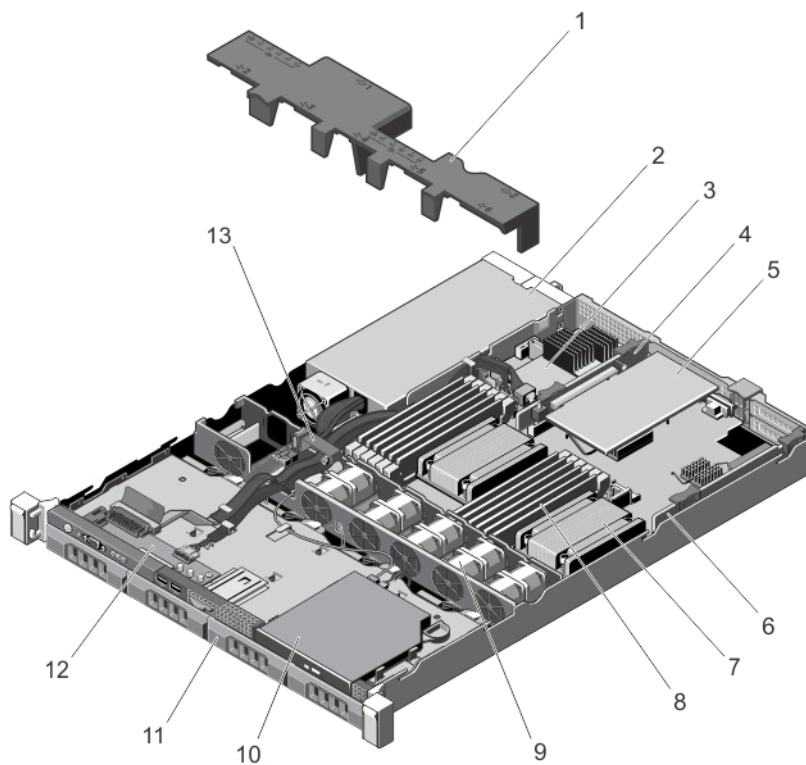
Abbildung 11. Innenansicht des Systems – mit einem nicht redundanten Netzteil
