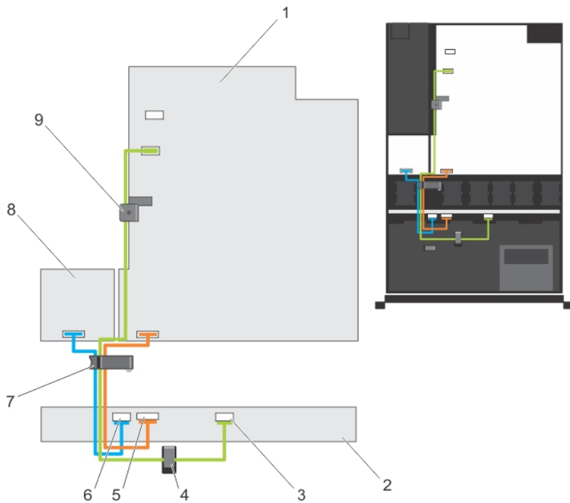
Abbildung 47. Diagramm zur Kabelführung – Rückwandplatine für vier Festplatten
