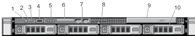
Abbildung 1. Merkmale und Anzeigen auf der Vorderseite – System mit vier 3,5-Zoll-Festplatten
