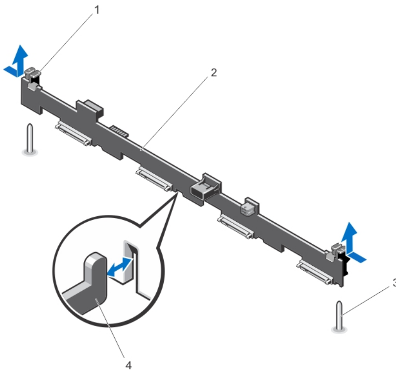
Abbildung 46. Rückwandplatine für vier Festplatten entfernen und installieren
