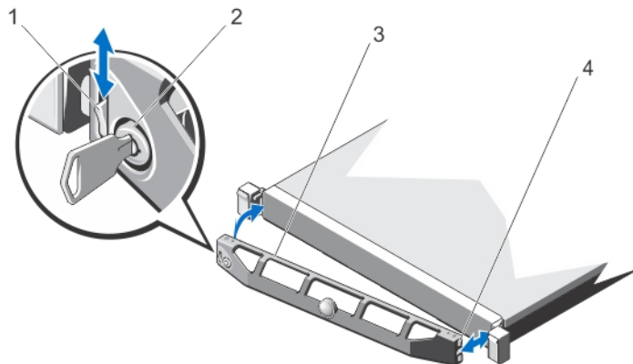
Abbildung 9. Frontverkleidung installieren und entfernen
