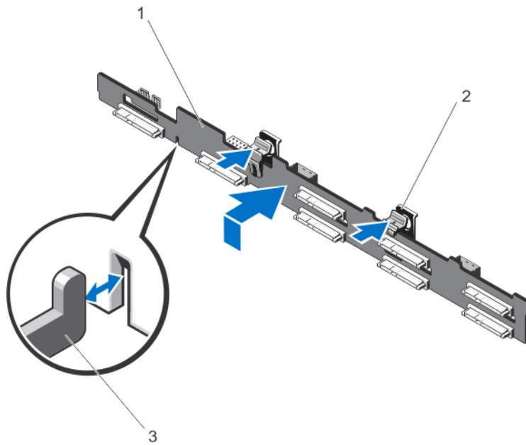
Abbildung 50. Rückwandplatine für acht Festplatten entfernen und installieren
