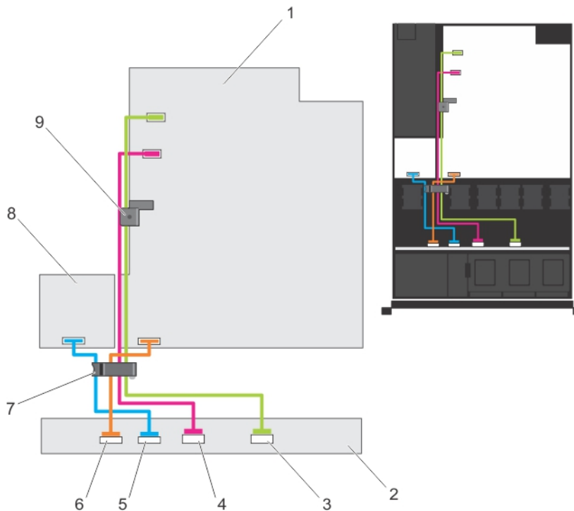
Abbildung 51. Diagramm zur Kabelführung – Rückwandplatine für acht Festplatten
