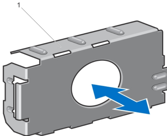
Abbildung 42. Netzteilplatzhalter entfernen und installieren
