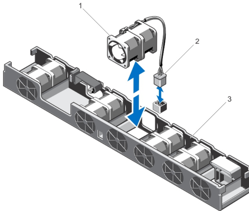
Abbildung 28. Lüfter entfernen und installieren
