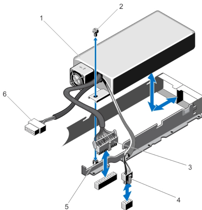
Abbildung 41. Nicht redundantes Netzteil entfernen und installieren
