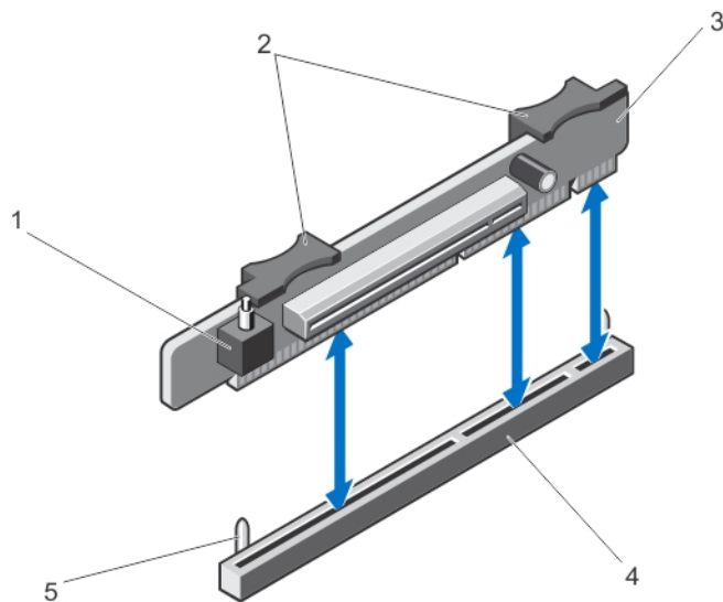
Abbildung 33. Entfernen und Installieren von Erweiterungskarten-Riser 2
