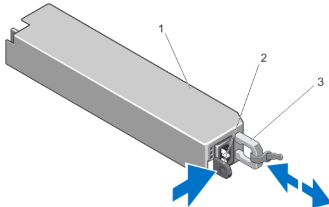
Abbildung 40. Redundantes Netzteil entfernen und installieren
