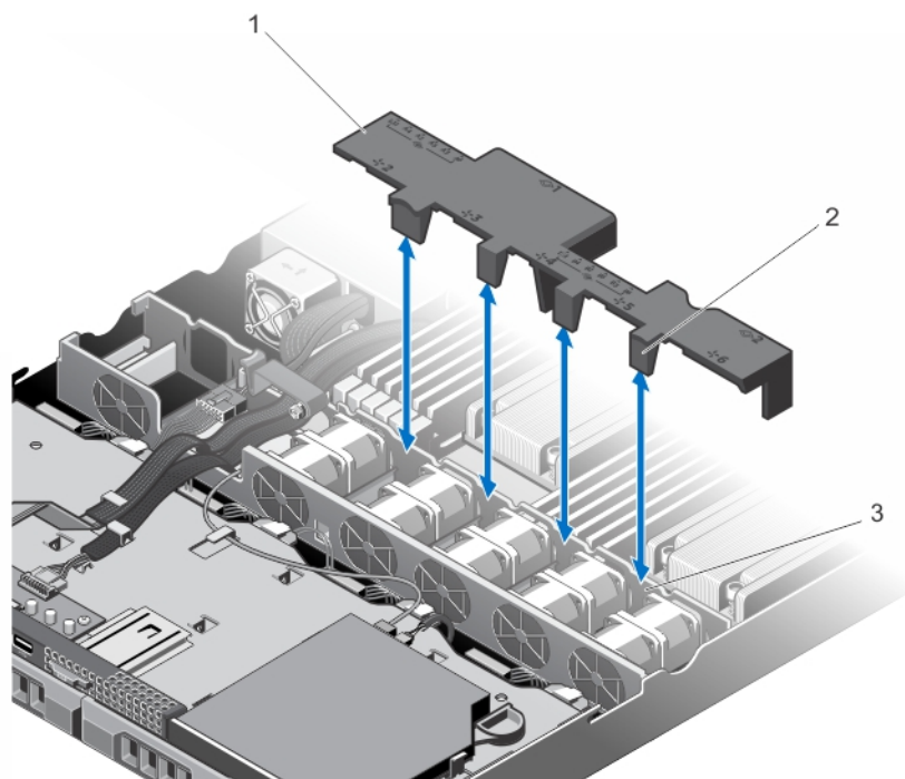
Abbildung 13. Kühlgehäuse entfernen und installieren
