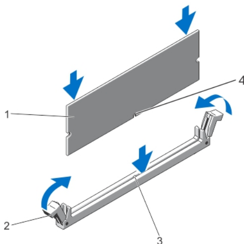
Abbildung 17. Einbauen des Speichermoduls
