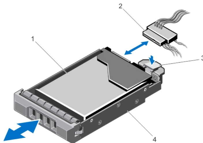
Abbildung 21. Verkabeltes Festplattenlaufwerk entfernen und installieren
