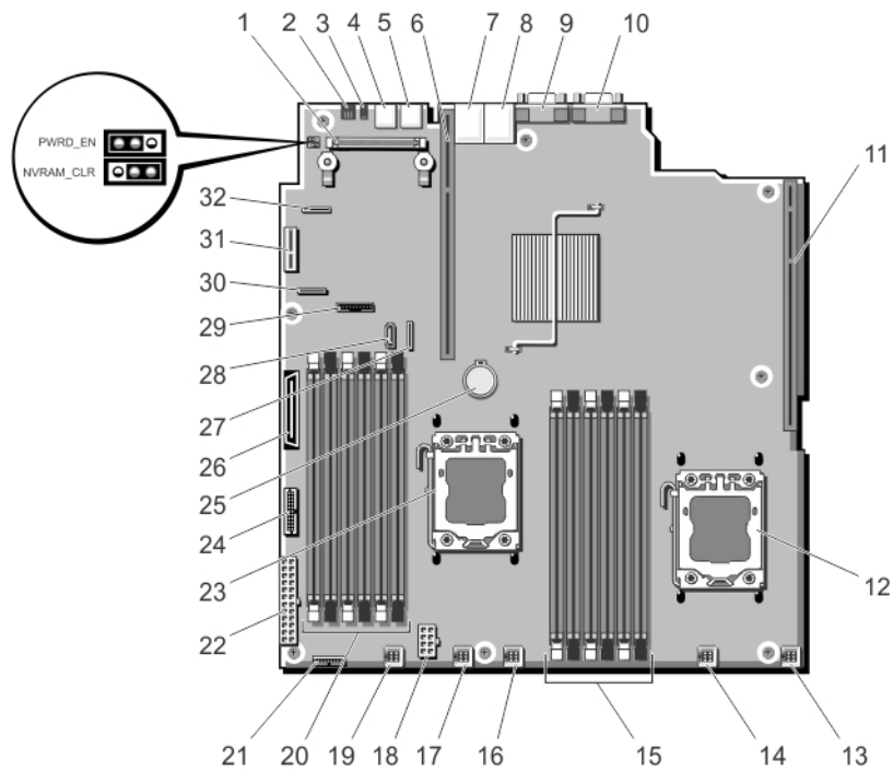
Abbildung 61. Jumper und Anschlüsse auf der Systemplatine
