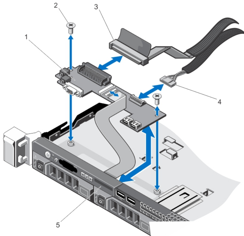
Abbildung 55. Bedienfeldmodul entfernen und installieren – System mit hot-plug-fähigen 3,5-Zoll-Festplatten
